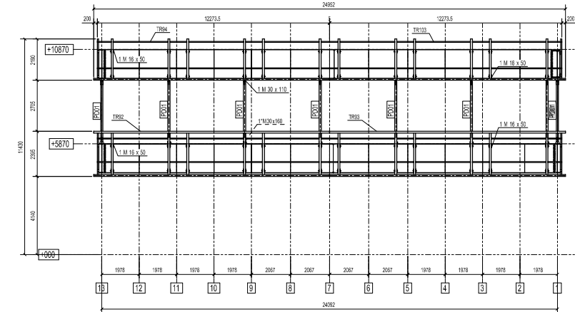
VISTA SU - FILO A
