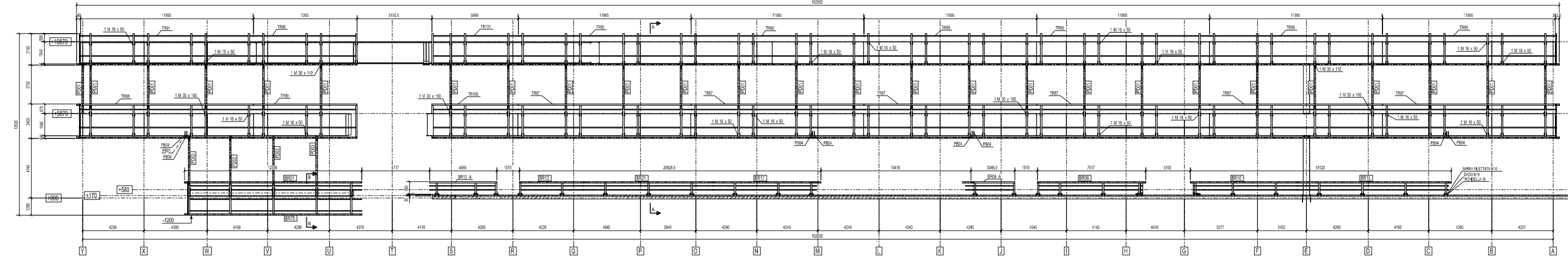
VISTA SU - FILO Y
