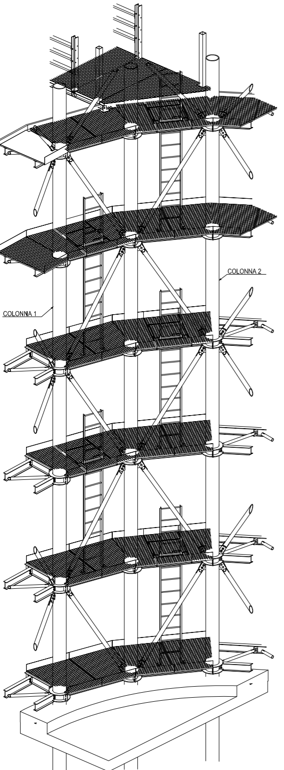
ASSONOMETRIA SCALE A PIOLI
