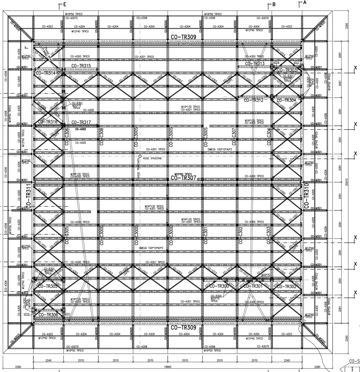
Pianta COPERTURA SCALA 1:50
