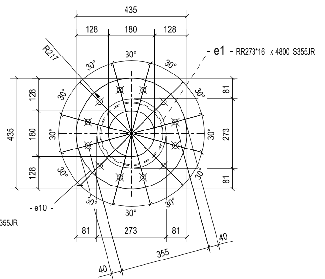
C - C
